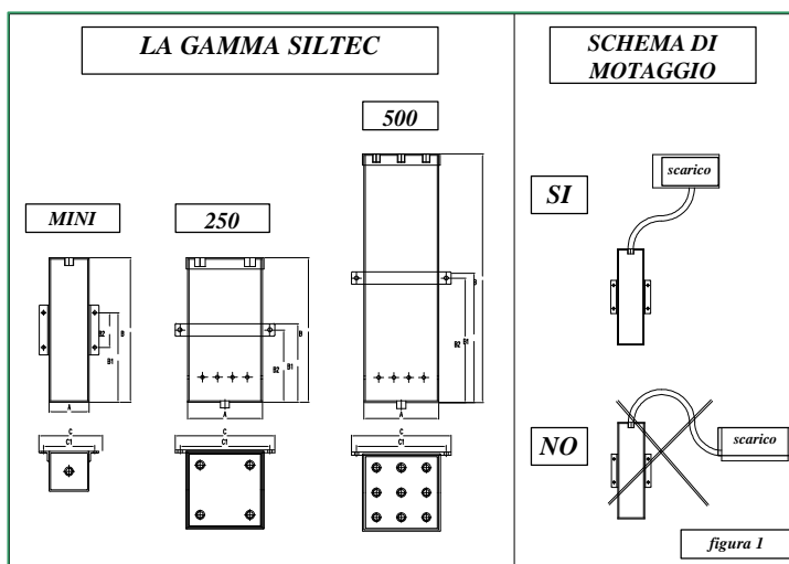
Alcuni modelli di silenziatori ad espansione SILTEC
